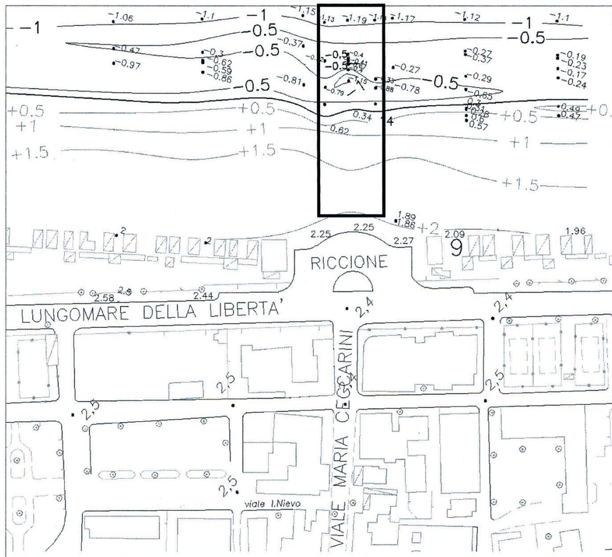
PLANIMETRIA SCALA 1:1000
