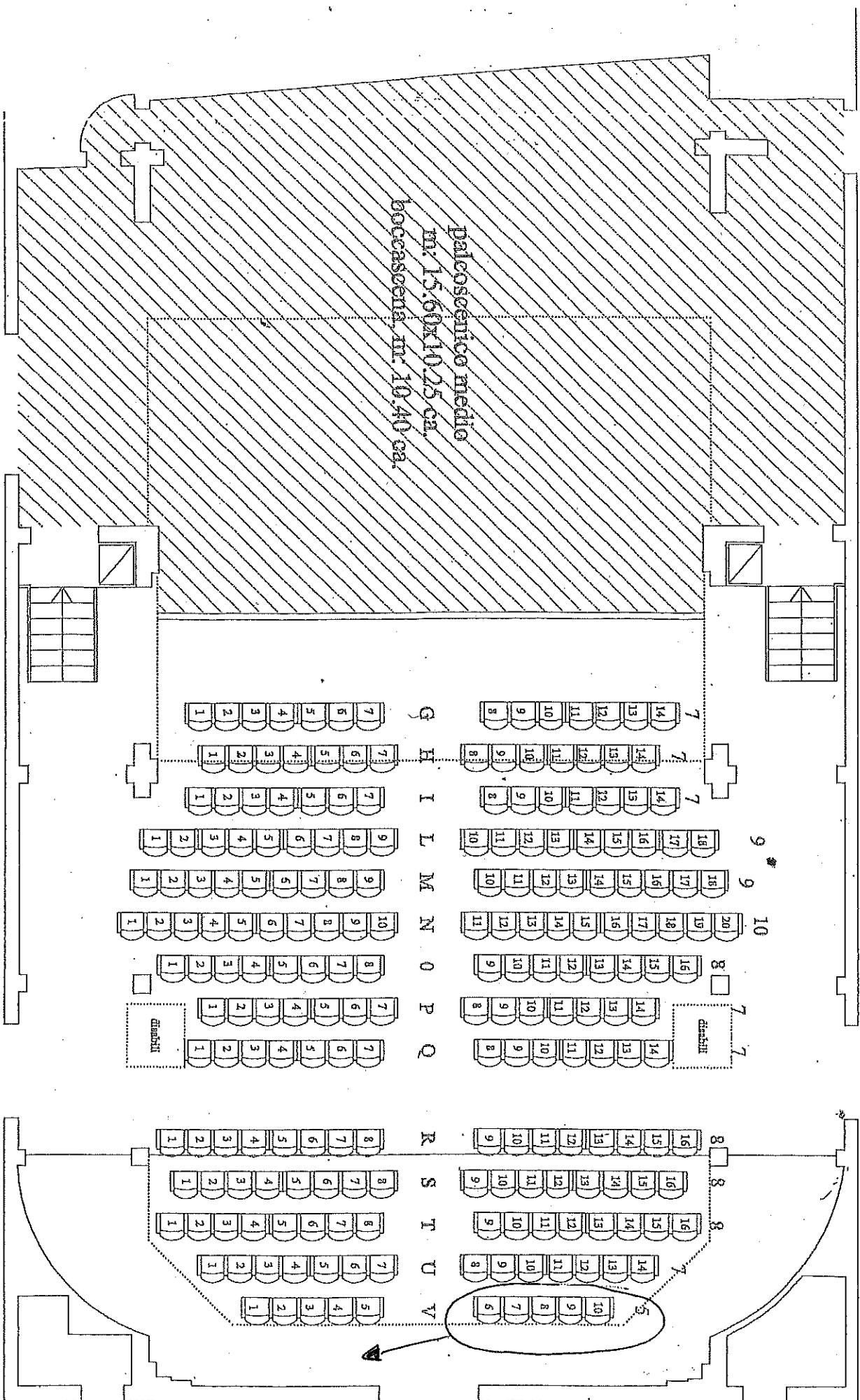
Soluzione palcoscenico medio: pianta della platea, 214 posti + 2 per disabili, scala 1:100
